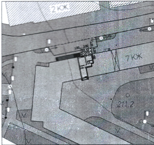
"Реконструкція квартири №108 під магазин промислових товарів та салон краси по вул. Шевченка, 2 в м. Фастів Київської області" Схема благоустрою прилеглої території М 1:500
